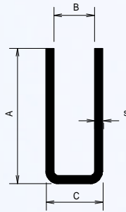
U-Laufnuten
