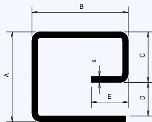
E2-Laufnuten
