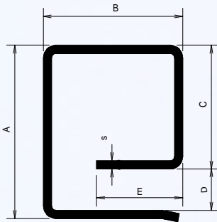
E1-Laufnuten
