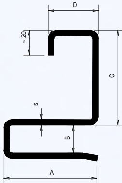
S-Laufnuten
