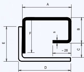
C-Laufnuten 2-tlg.
