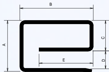
C-Laufnuten
